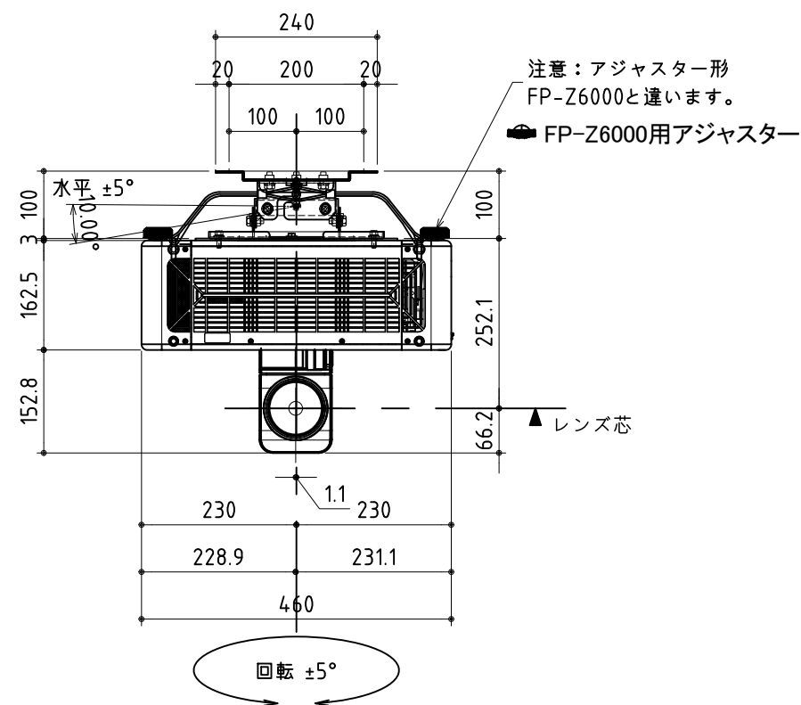
正面図
