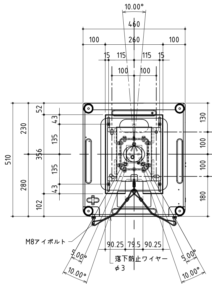
平面図
