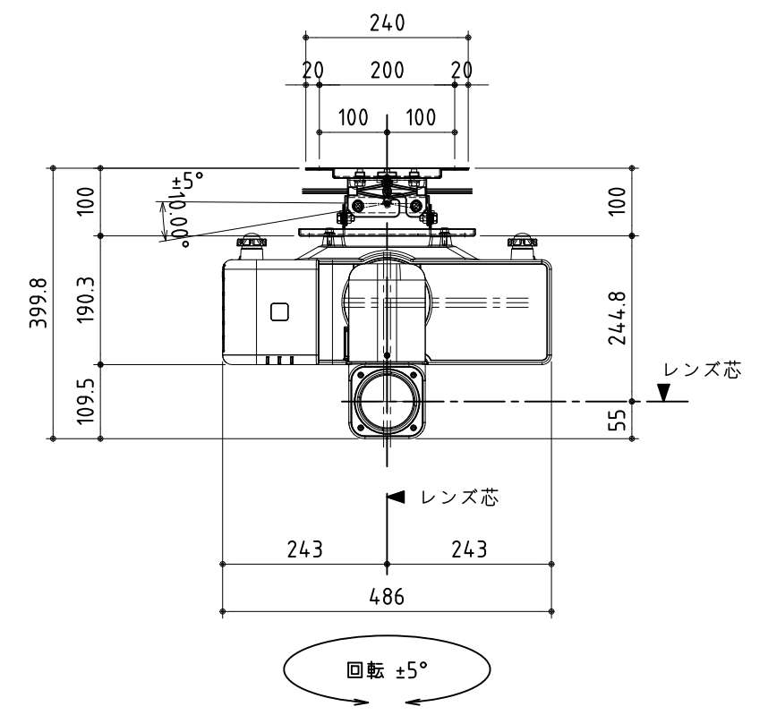
正面図
