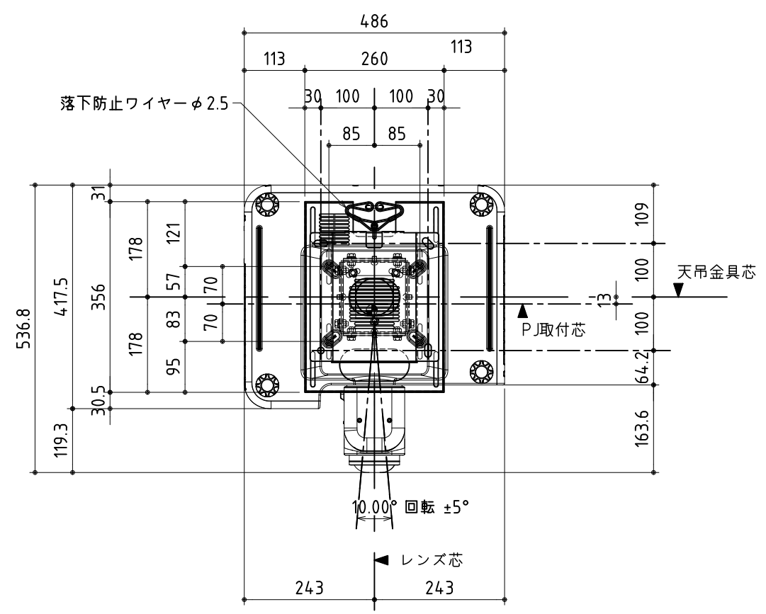
平面図
