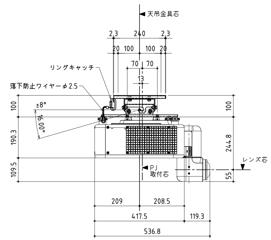
側面図
