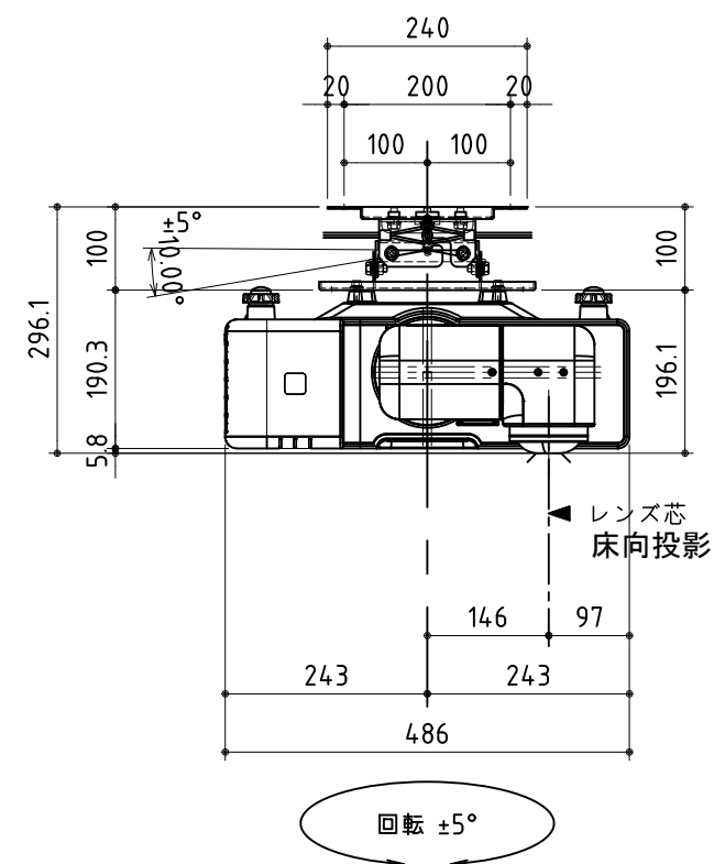
正 面 图
