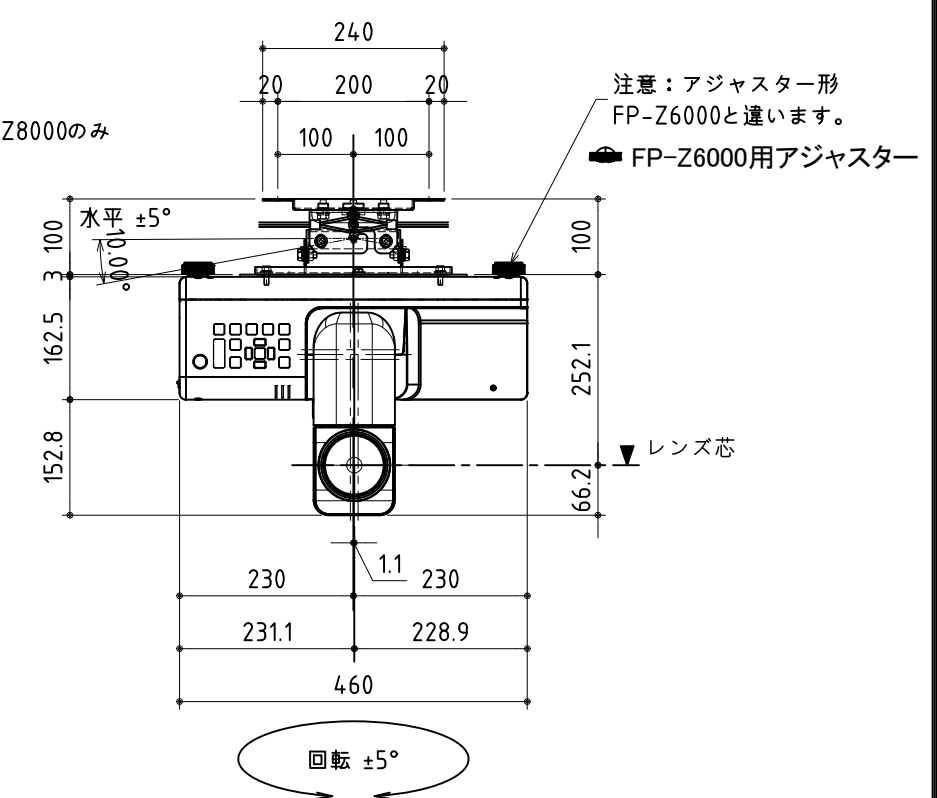
正面図
