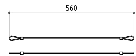
落下防止ワイヤー φ3 FP-Zシリーズ用(2本) この機種に使用します。
