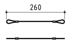
落下防止ワイヤー φ2.5 FP-ZUHシリーズ用(2本)
