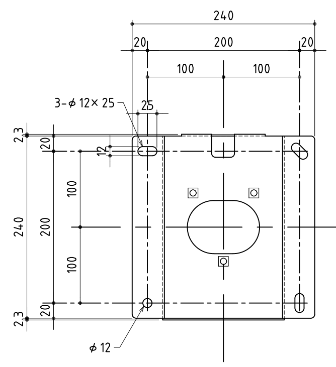
天井取付金具伏図 1/5
