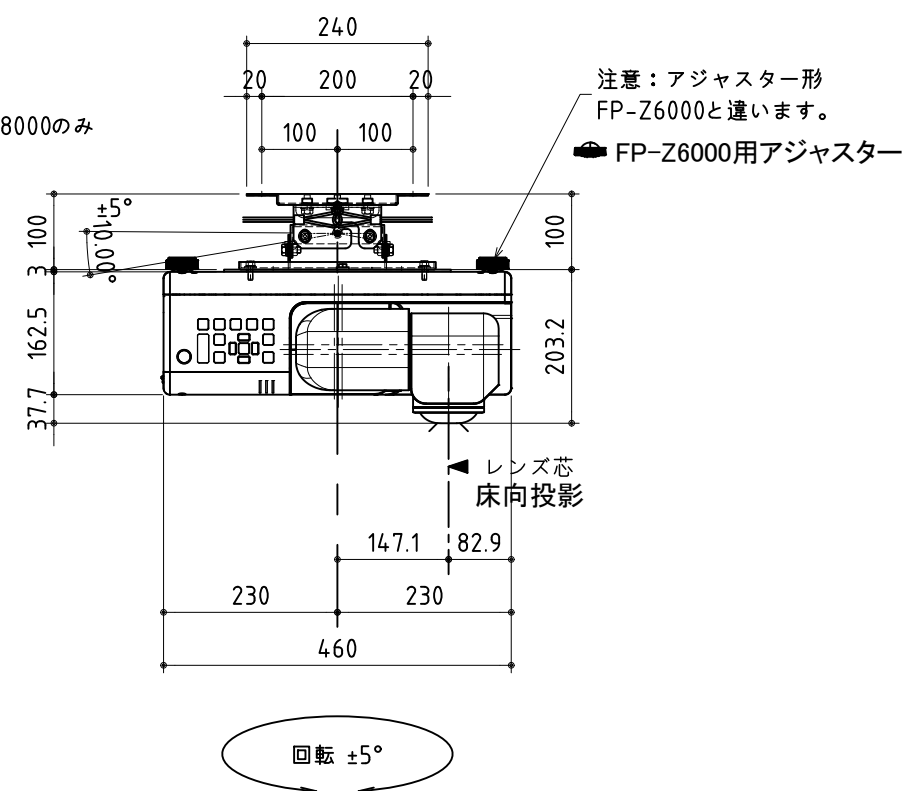
正面図
