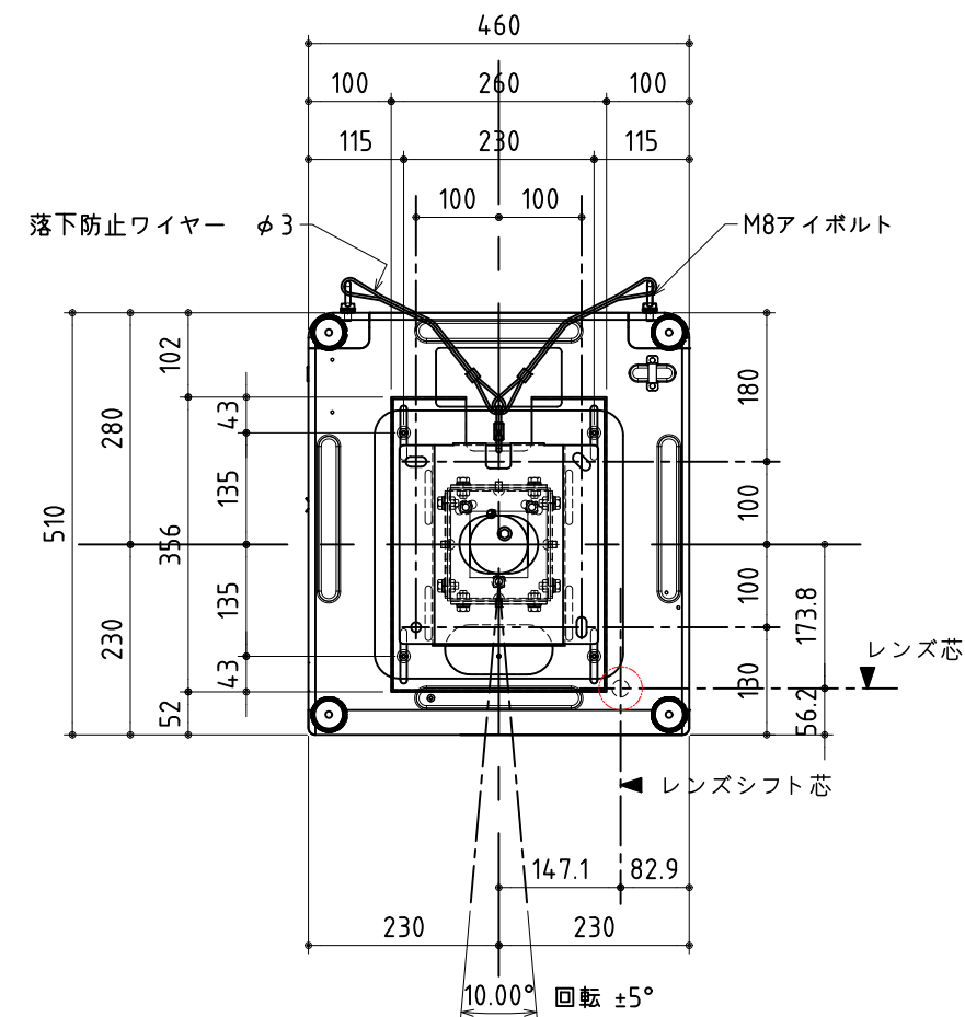
平面図
