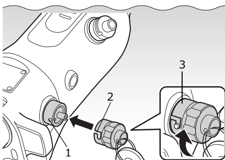
1: ピン 2: 切り欠き 3: タンク受けキャップ
